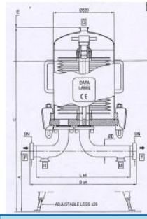
Filtere lenticulaire à modulee
