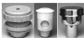
Soupapes pression/dépression Existe aussi pour milieu ATEX
