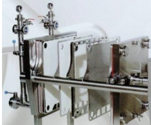
Filtere presse : 40x40-50x50-60x60 Existe en version étanche
